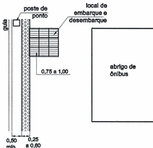
Figura 74 — Sinalização tátil no ponto de ônibus – Exemplo
