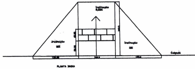
RAMPA PARA REBAIXAMENTO DO TIPO A
