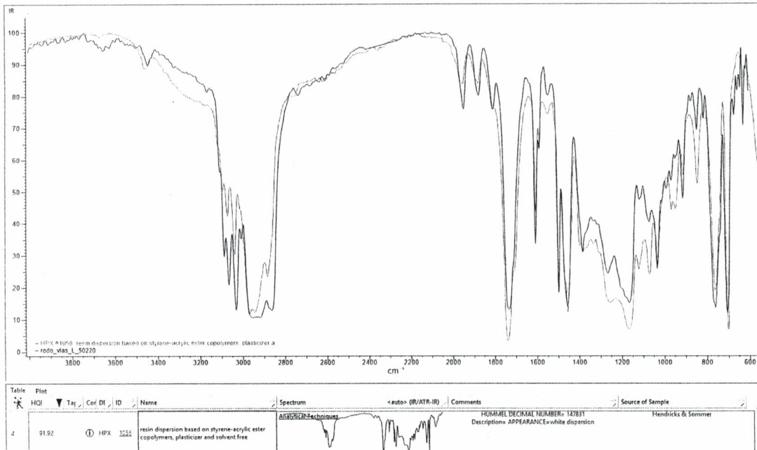
Espectrograma de infravermelho da resina da tinta
