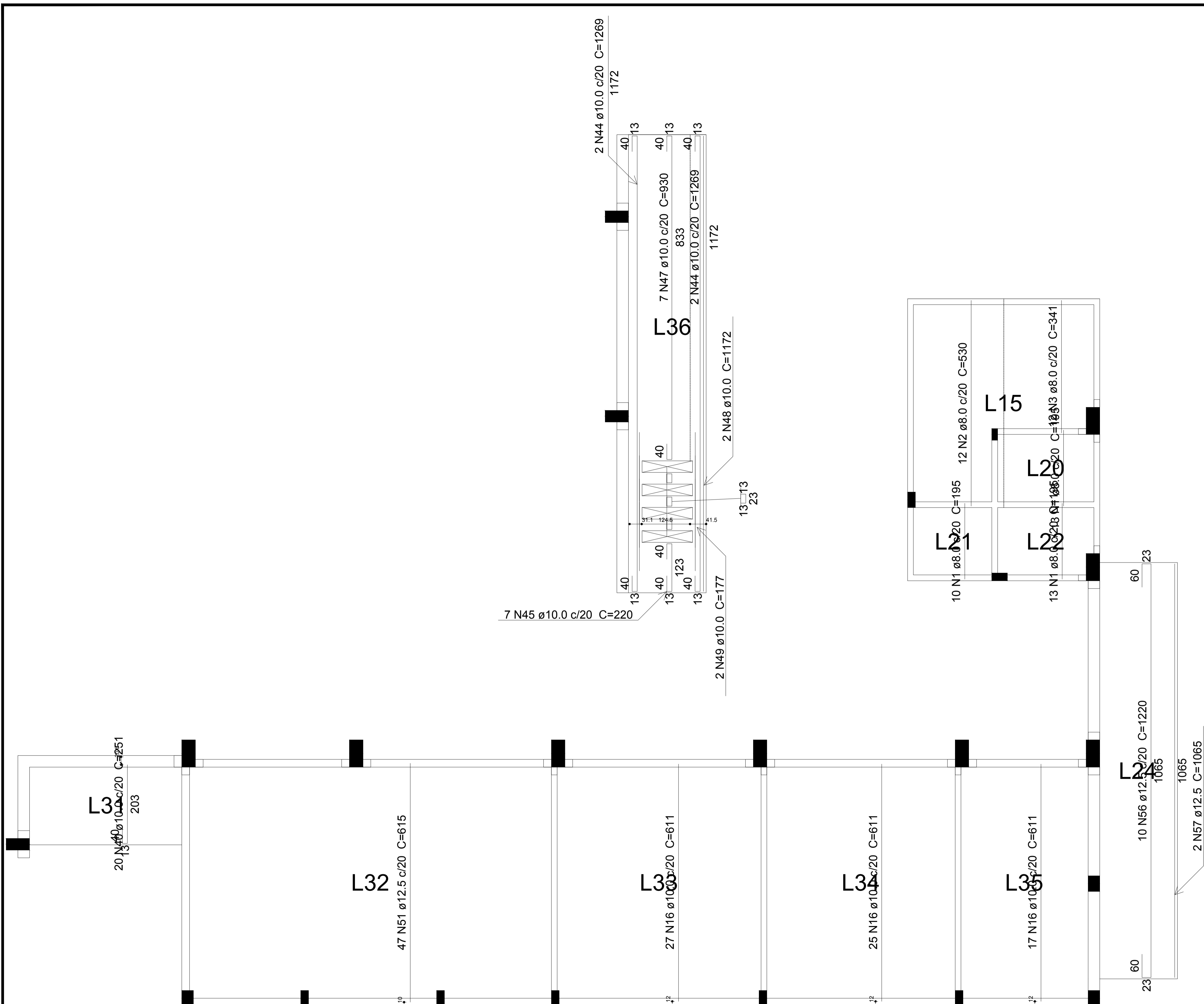
28 ARMAÇÃO POSITIVA DAS LAJES (EIXO Y) ESCALA: 1/50
