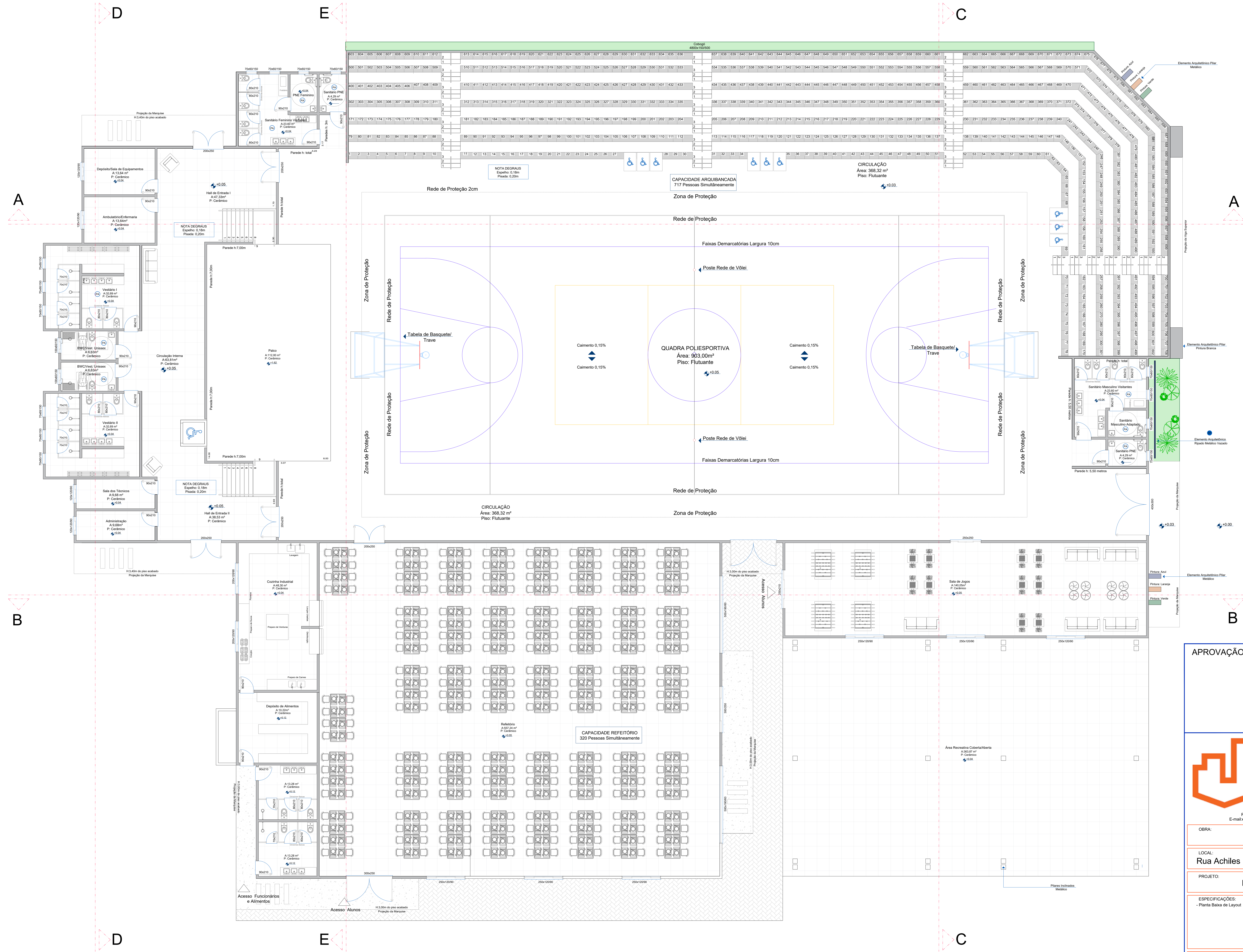
PLANTA DE LAYOUT Esc: 1/80
