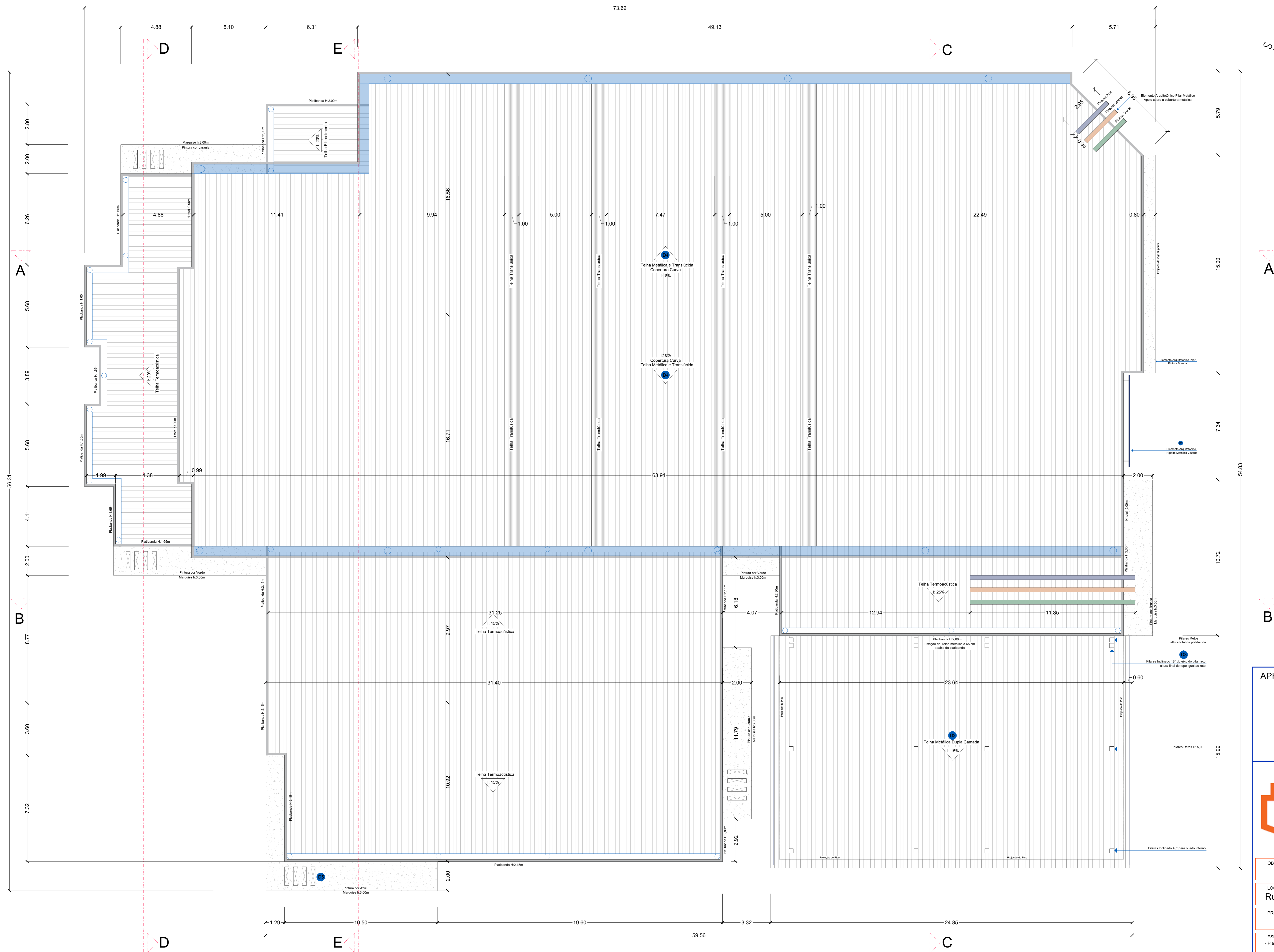
PLANTA DE COBERTURA Esc: 1/90
